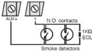
2-καλωδίων εγκατάσταση Κλέμες Πίνακα Ελέγχου
