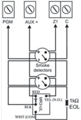
4-καλωδίων εγκατάσταση Κλέμες Πίνακα Ελέγχου
